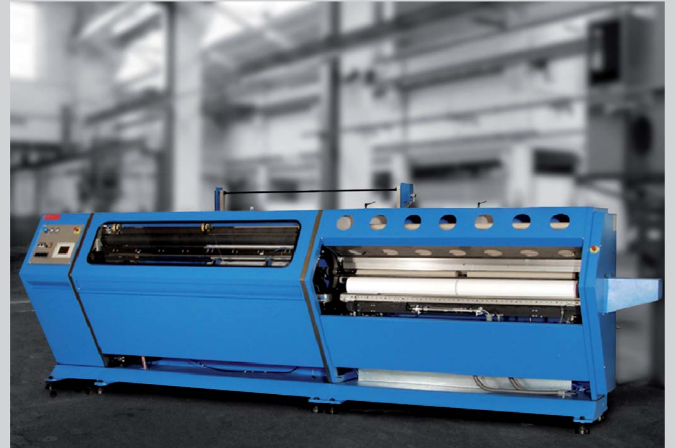
Parmi d'autres produits, la PW300 de GOEBEL fabrique des rouleaux de papier cadeau de façon totalement automatique. Dans un seul process, plusieurs largeurs de rouleaux peuvent être produites.
