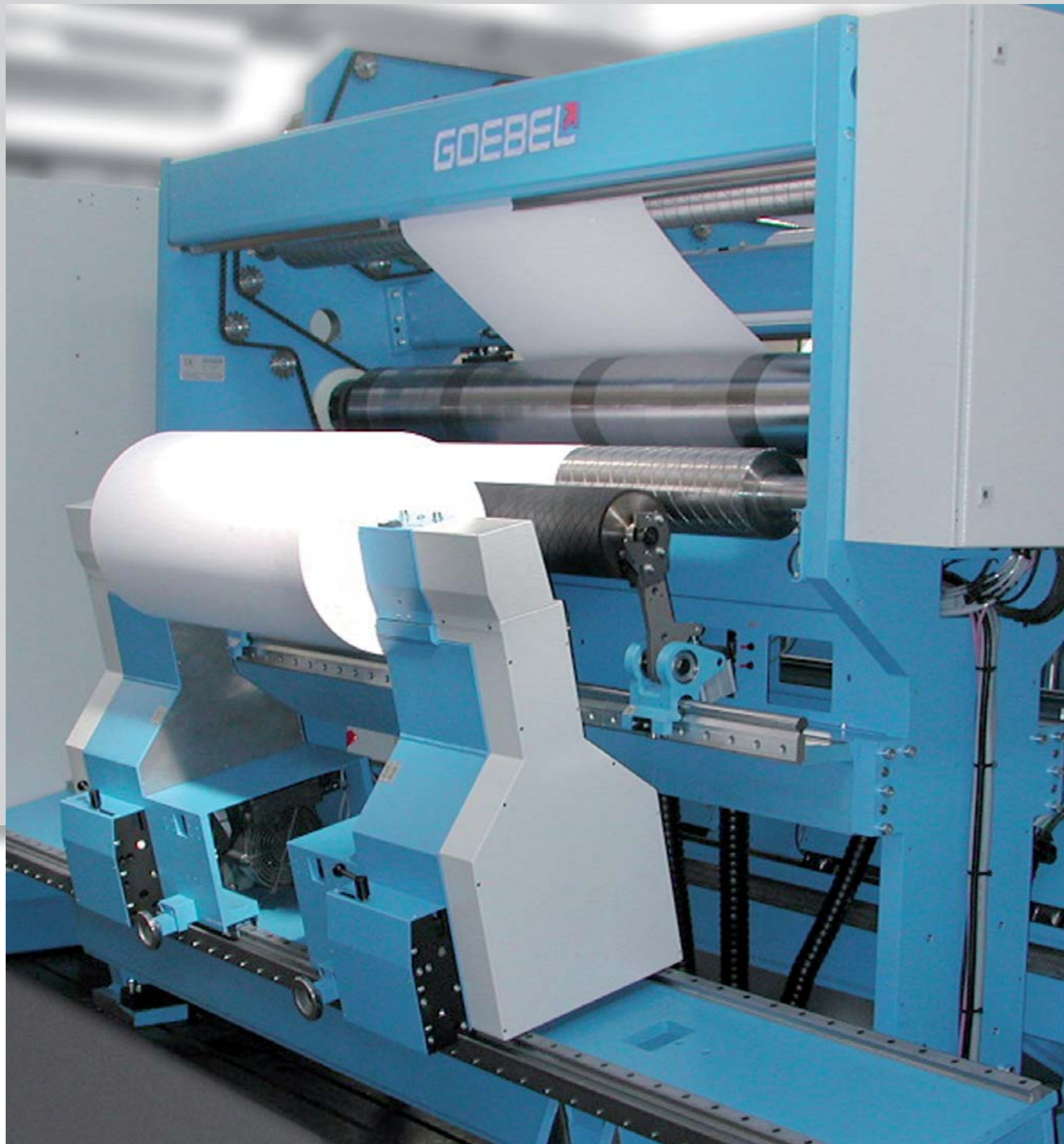
La machine xtraslit de GOEBEL avec enroulage central convertit tous les types de papier à une vitesse de marche pouvant atteindre 1 200 m/min.
